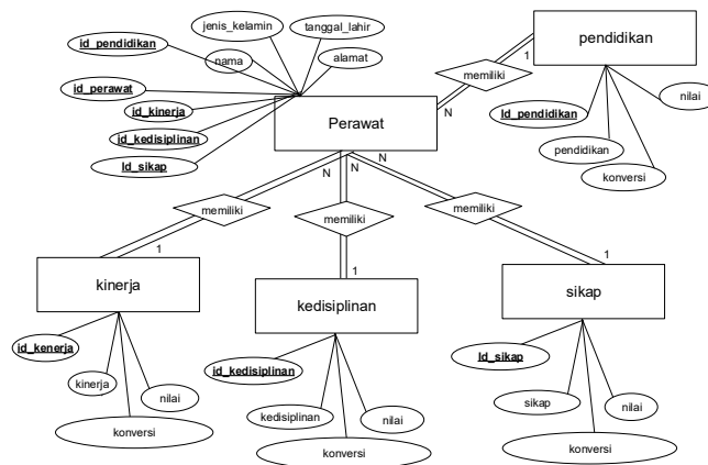
Gambar 5. ERD SPK Pemilihan Perawat
