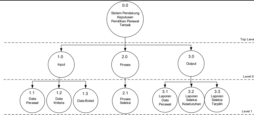
Gambar 3. Desain HIPO SPK Pemilih Perawat
