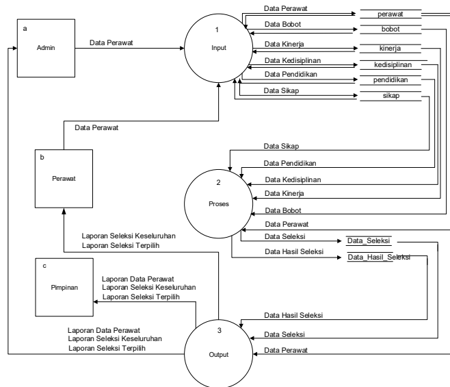
Gambar 4. DAD SPK Pemilihan Perawat
